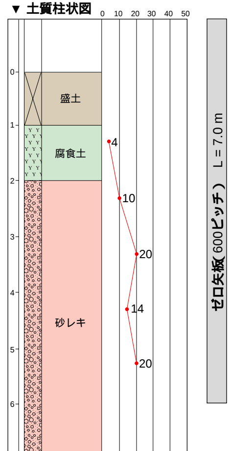
▼ 土質柱状図
