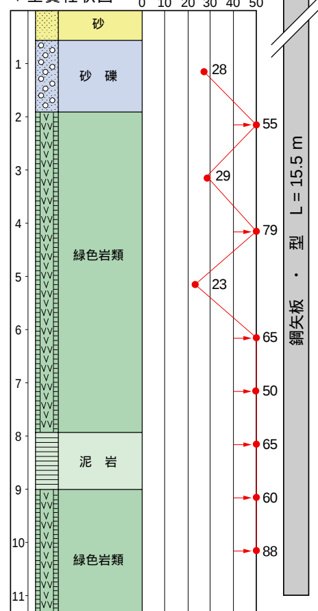
▼ 土質柱状図
