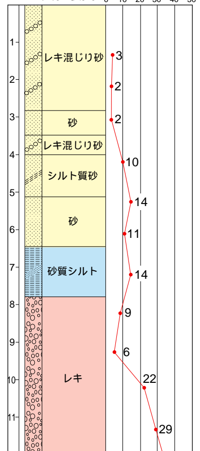
土質柱状図
