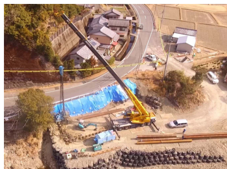
施工中(空中写真)
