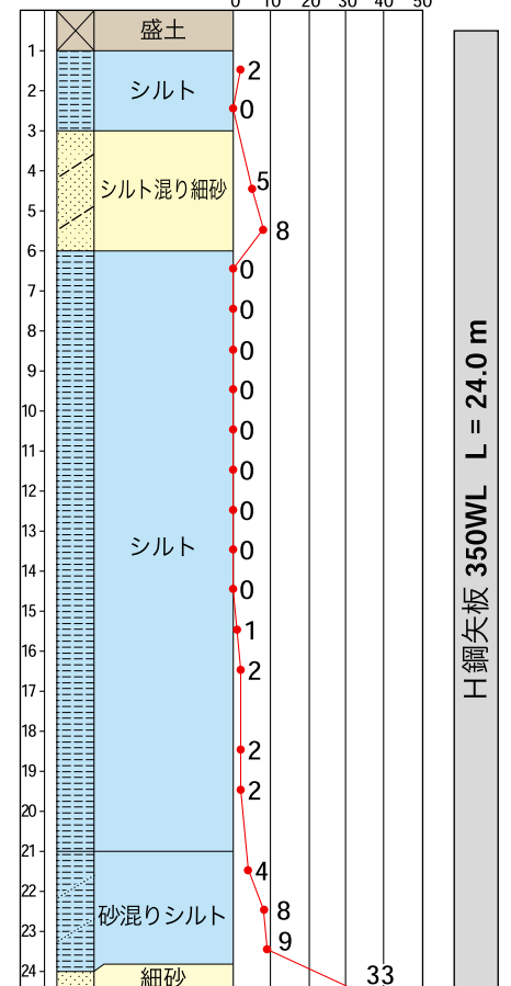
▼ 土質柱状図
