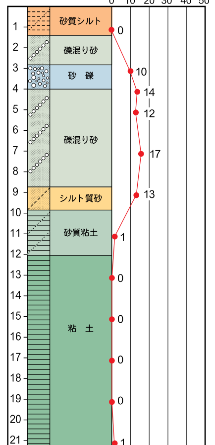
▼土質柱状図
