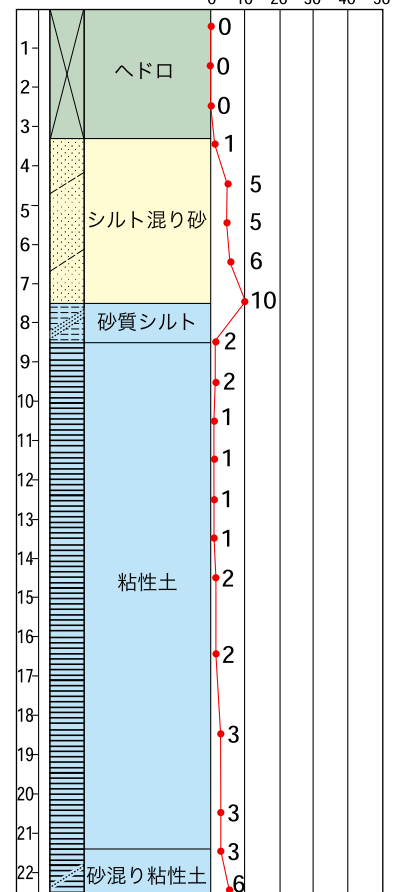
▼ 土質柱状図
