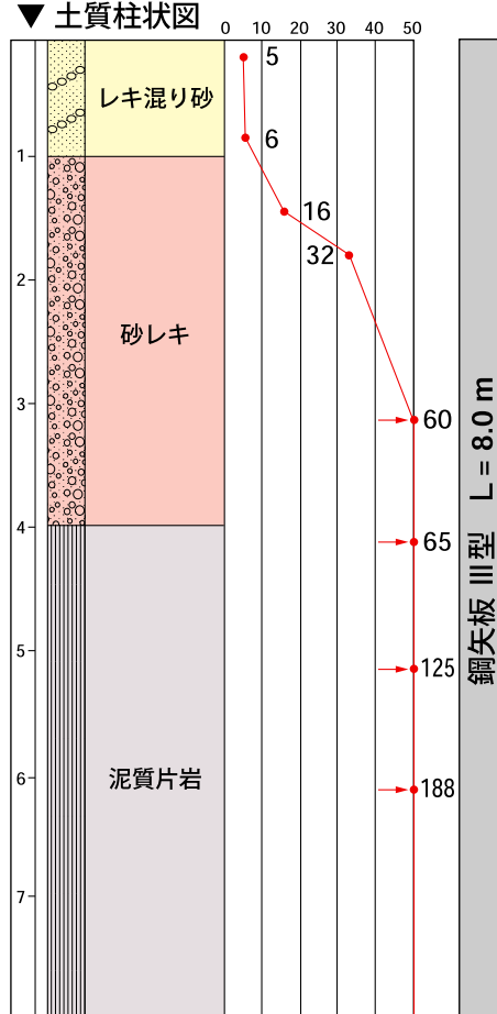
▼ 土質柱状図
