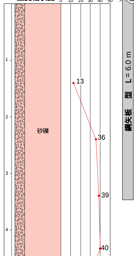
▼ 土質柱状図
