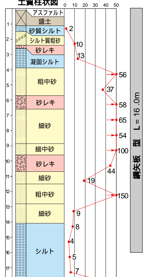
土質柱状図
