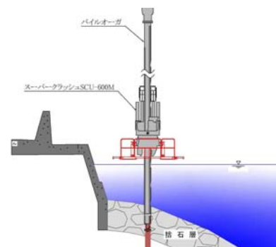
▲施工断面図
