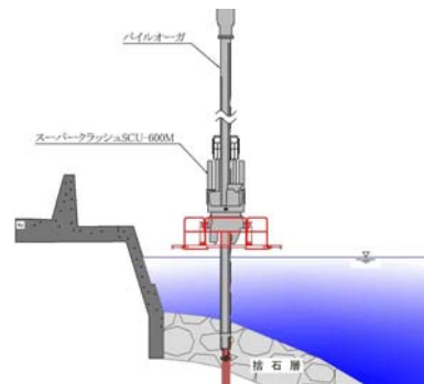
▲施工断面図
