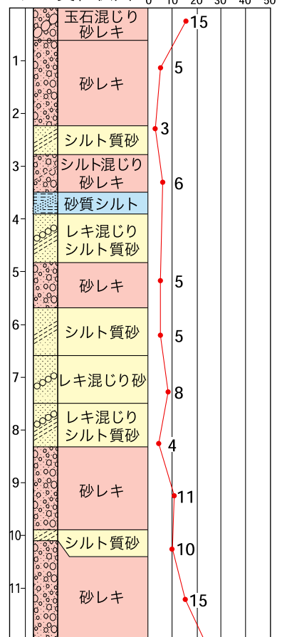
▼ 土質柱状図
