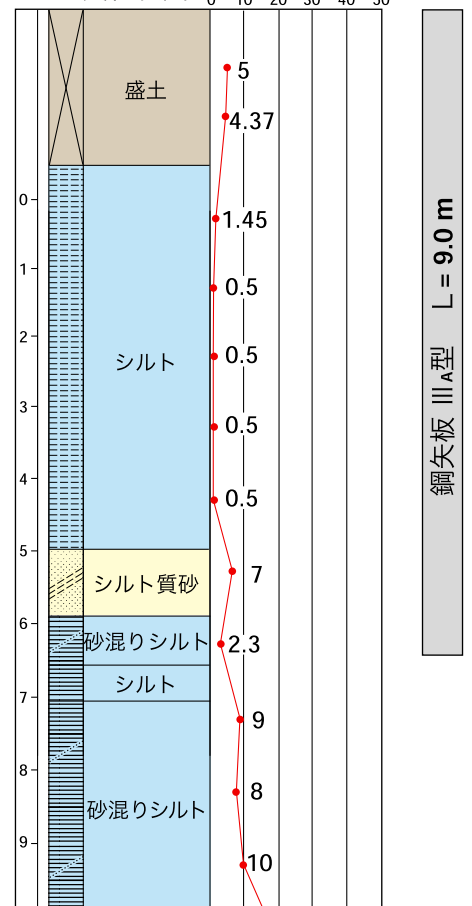
▼ 土質柱状図
