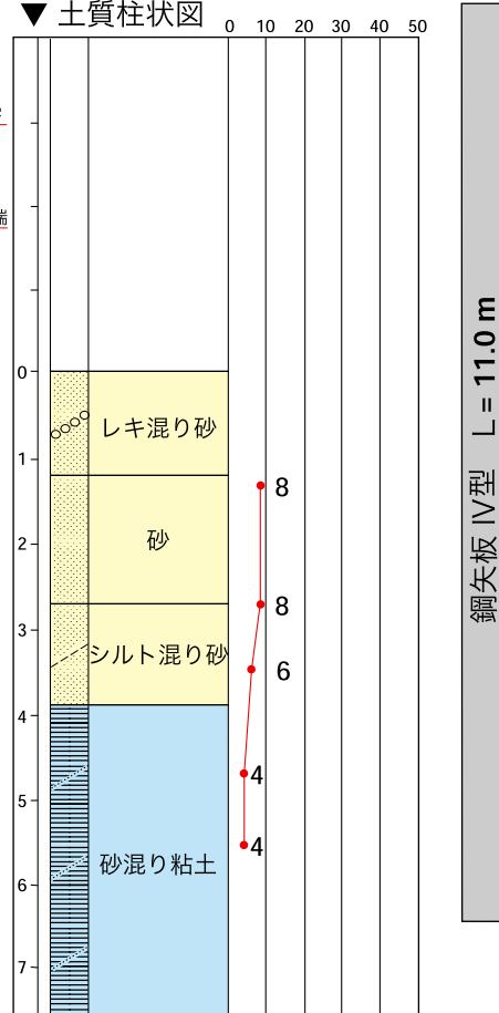
▼ 土質柱状図
