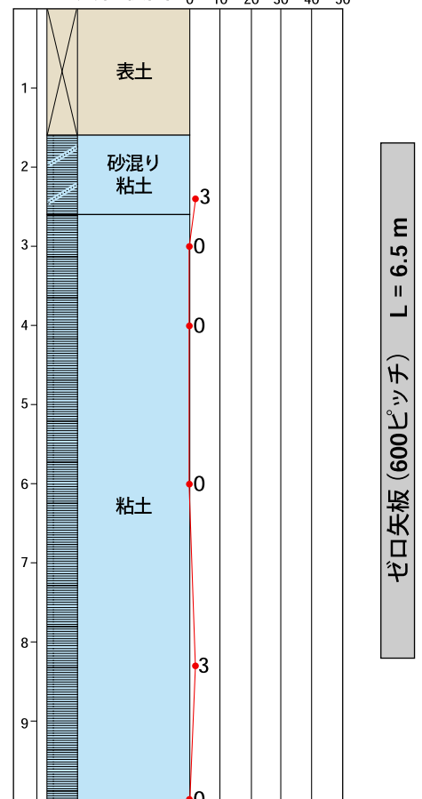
▼ 土質柱状図
