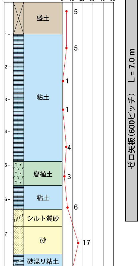
▼ 土質柱状図
