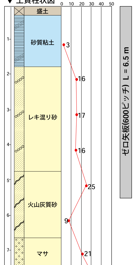
▼ 土質柱状図
