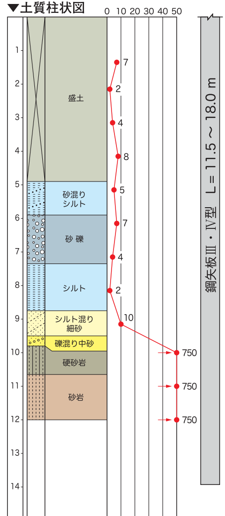
▼土質柱状図
