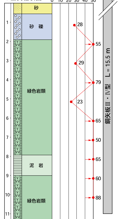
▼土質柱状図
