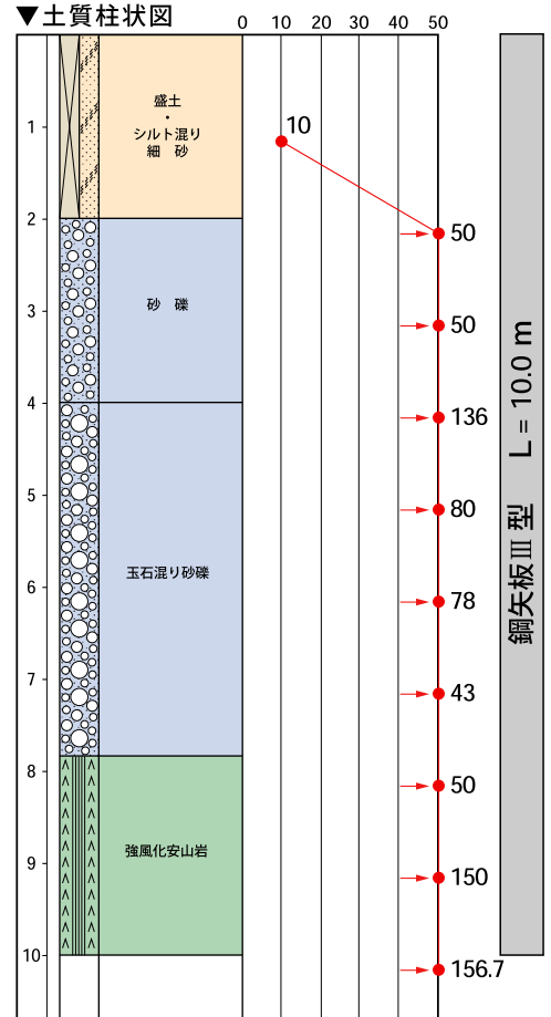
▼土質柱状図
