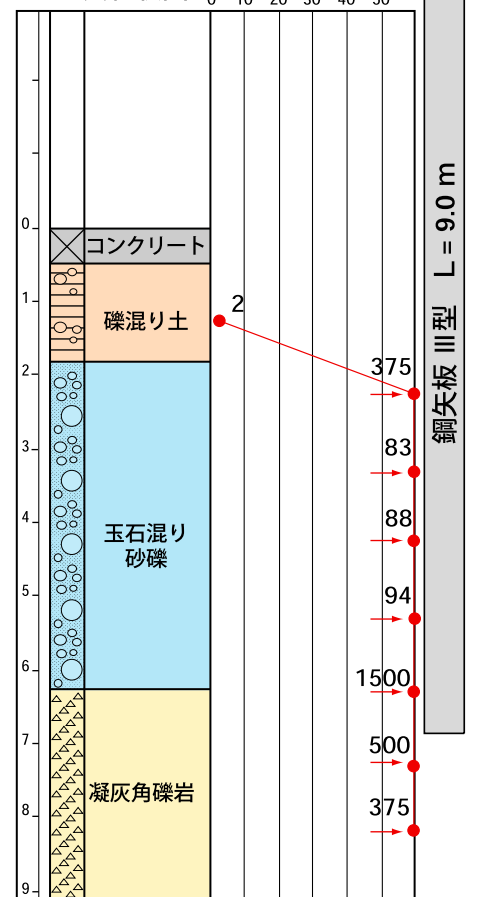
▼ 土質柱状図
