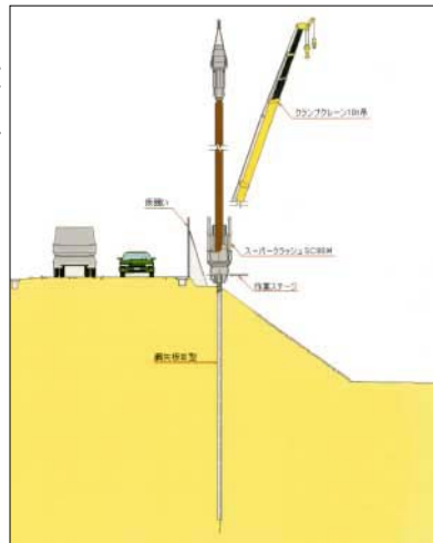
▶ 施工断面図
