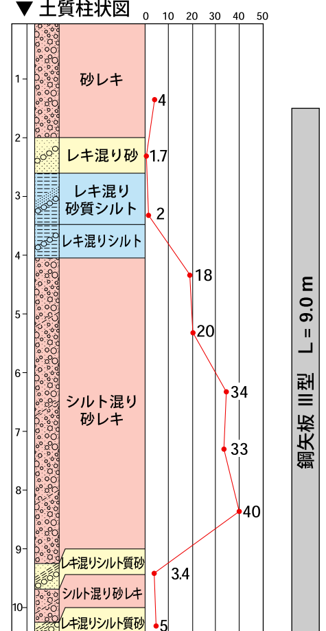
▼ 土質柱状図
