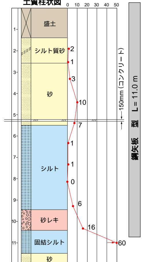
土質柱状図
