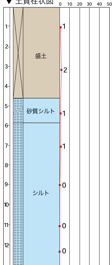
▼ 土質柱状図
