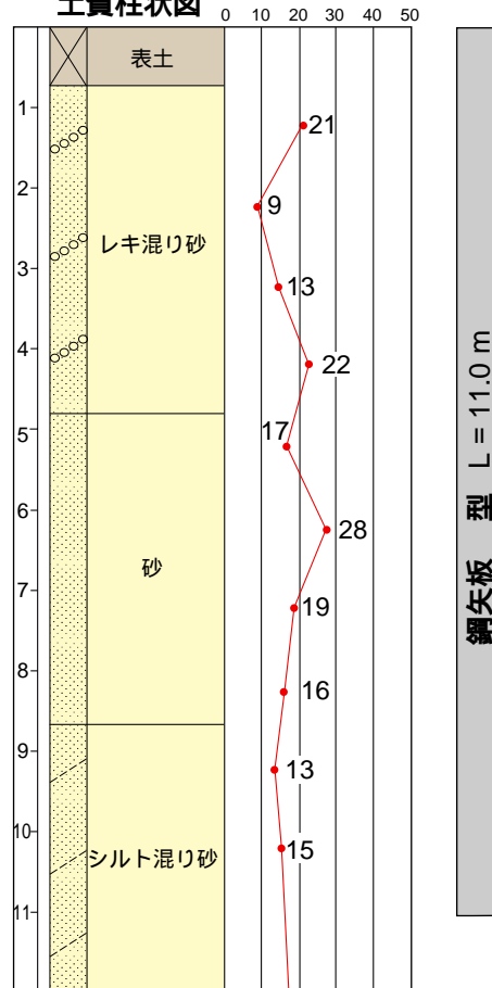
土質柱状図
