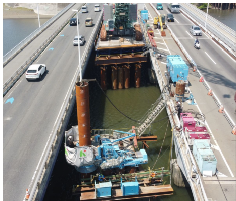
鋼管杭施工状況
