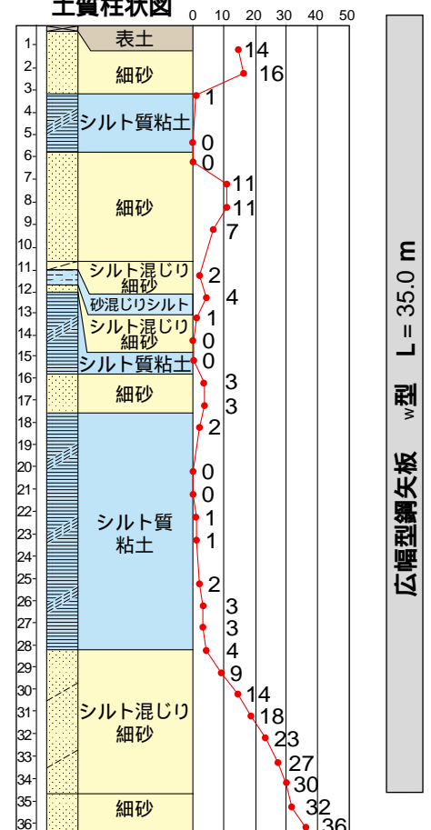
土質柱状図
