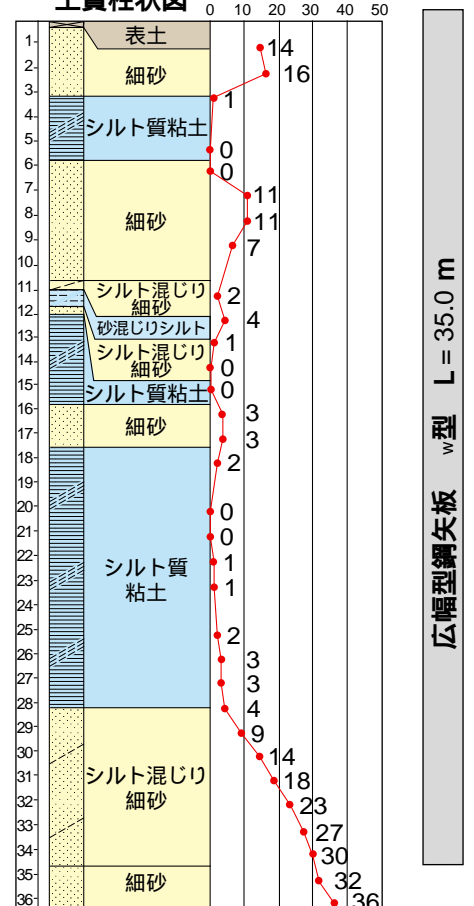
土質柱状図
