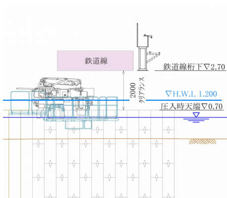
施工時断面図
