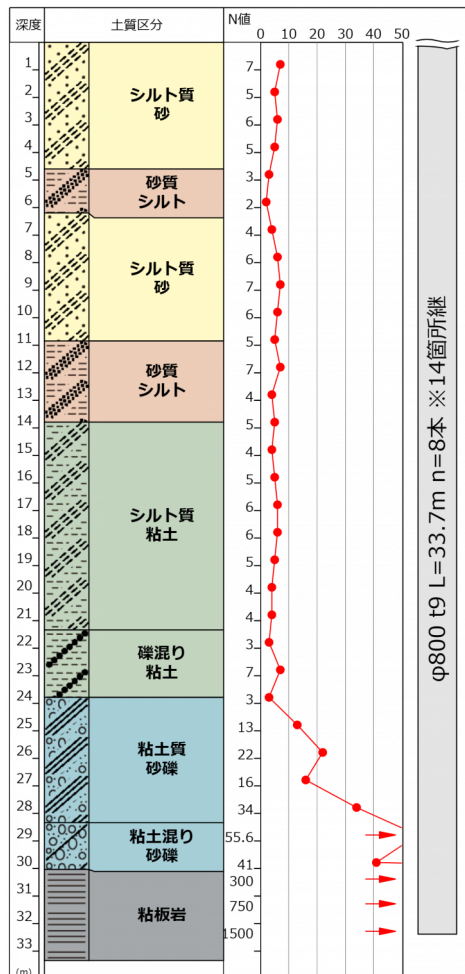
断面図
