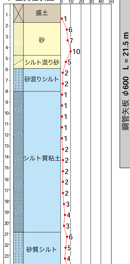
▼ 土質柱状図
