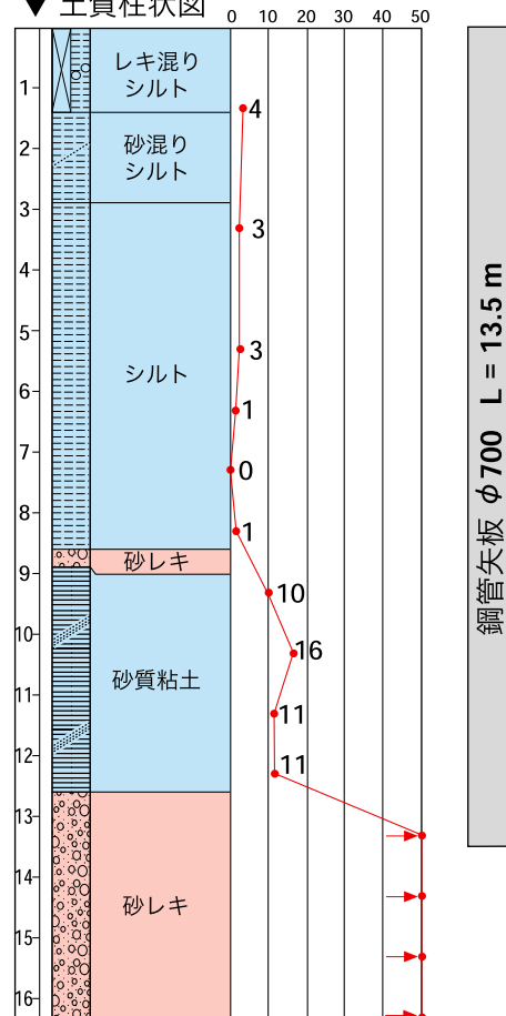
▼ 土質柱状図
