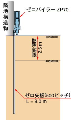
▼ 断面図
